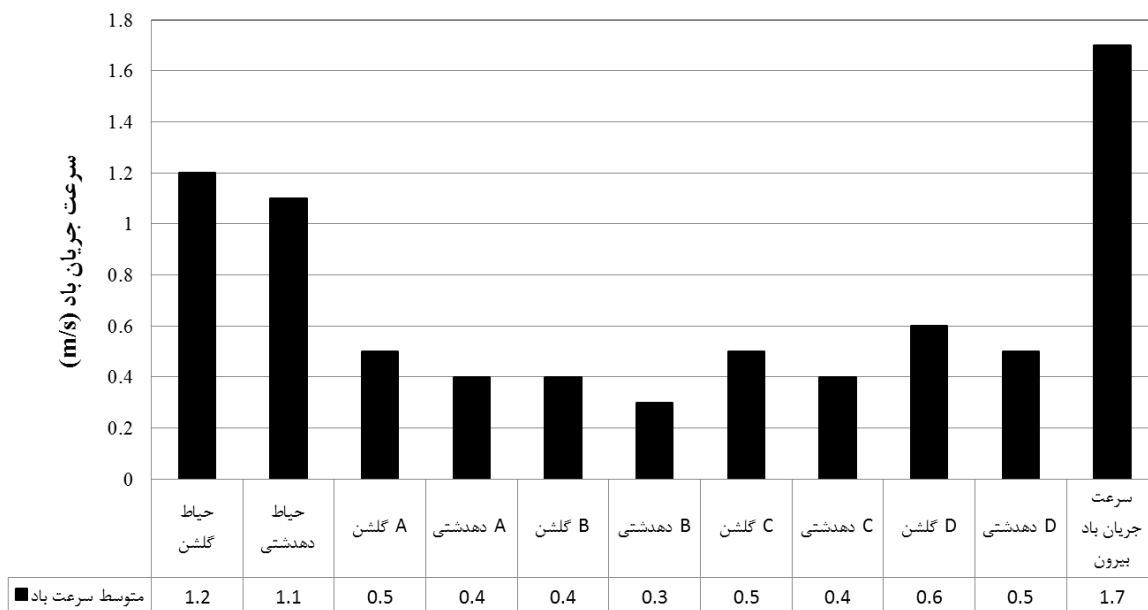
تصویر ۱۰- مقایسه ی متوسط سرعت جریان باد اندازه گیری شده در عمارت های دهدشتی و گلشن در روزهای آزمون، ۱۳۹۵.
