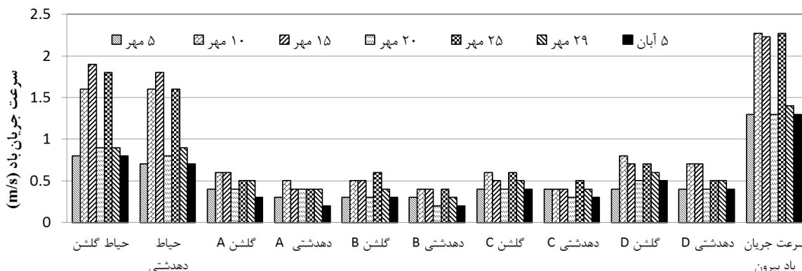
تصویر ۹- مقایسه ی سرعت جریان باد اندازه گیری شده در عمارت های دهدشتی و گلشن در روزهای آزمون، ۱۳۹۵.
