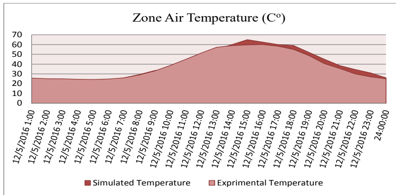
نمودار ۷- نمودار مقایسه دمای درونی نمونه شبیه سازی شده با نمونه ساخته شده گلخانه خورشیدی در ۲۴ ساعت اول.
