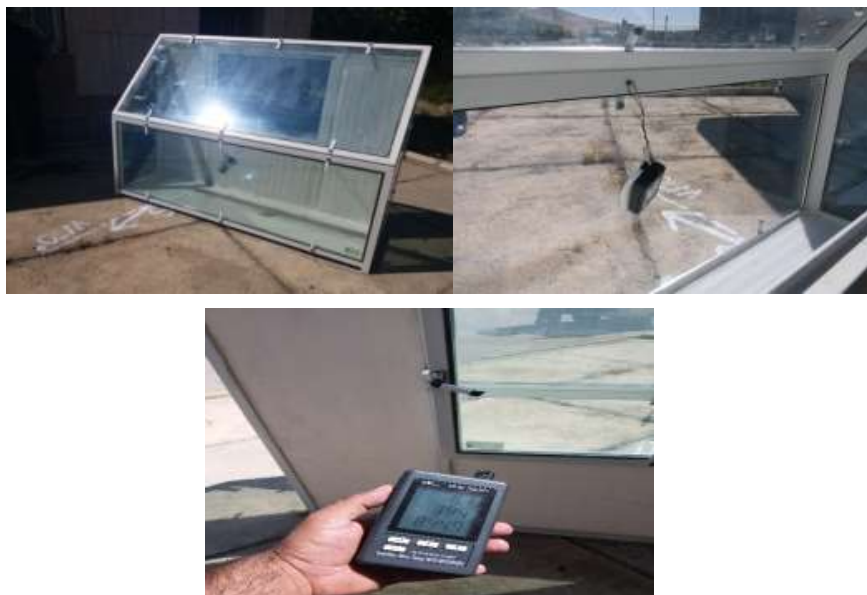
تصویر ۷- درز بندی و موقعیت نصب دستگاه دیتالاگر در درون نمونه ساخته شده گلخانه خورشیدی و چرخش برای دریافت حداکثر تابش خورشیدی.
