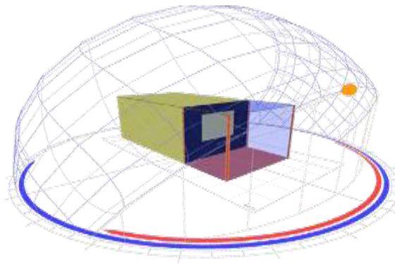
تصویر ۲- مدل شبیه‌سازی شده در نرم‌افزار انرژی پلاس.
