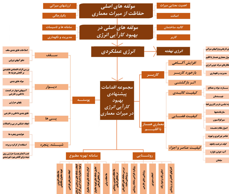
تصویر ۶- مجموعه اقدامات پیشنهادی بهبود کارایی انرژی در بناهای تاریخی.
