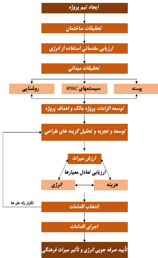
تصویر ۵- روندنمای برنامه ریزی و اجرای پروژه به سازی انرژی بنای تاریخی. مأخذ: (Hayter et al., 2019, 29)
