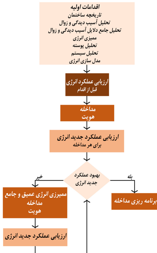
تصویر ۲- روندنمای اقدامات بهینه سازی مصرف انرژی، انجمن ایتالیایی تهویه مطبوع، گرمایش و سرمایش. مأخذ: (Franco & Magrini, 2017, 51)
