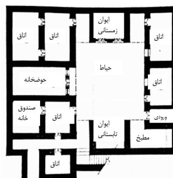
تصویر ۳- سمت راست: نمونه‌ای از پلان یک خانه مسکونی در فردوس قدیم. برای مقابله با زلزله، ۱۳۷۳، ۶۶
