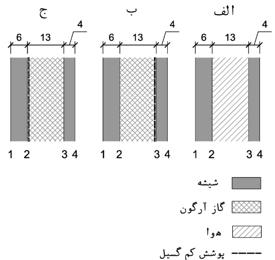
تصویر ۱ - الف: شیشه دوجداره ساده.
