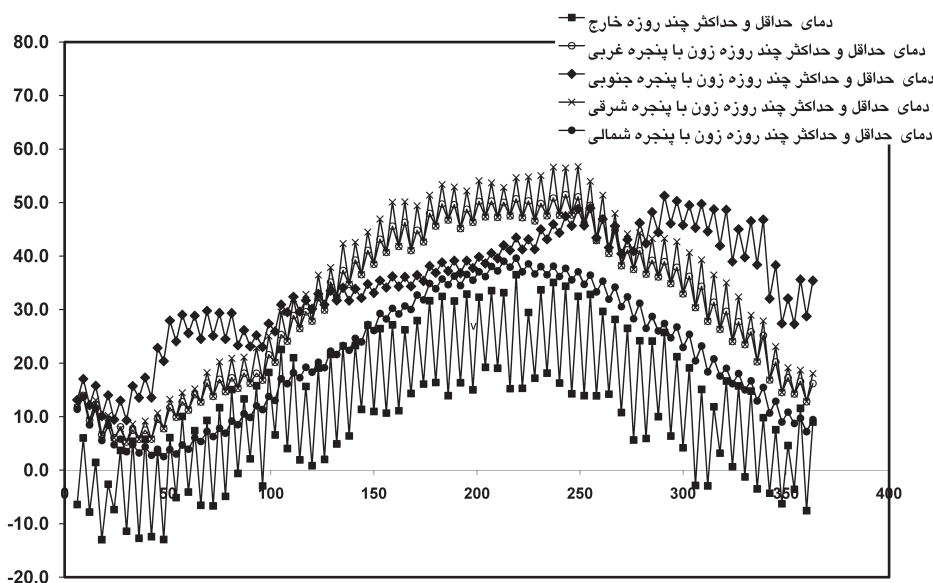
تصویر ۱۲ - دمای (حدافل و حداکثر) هوای خارج و داخل فضای بدون تهویه، در صورت کاربرد شیشه تک‌جداره ساده در چهار جهت اصلی ساختمان در شهراردییل.
