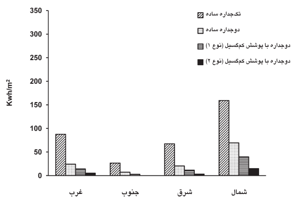
تصویر ۱۰ - بار حرارتی شیشه‌های مورد مطالعه در اوقات سرد سال در چهار جهت اصلی ساختمان.
