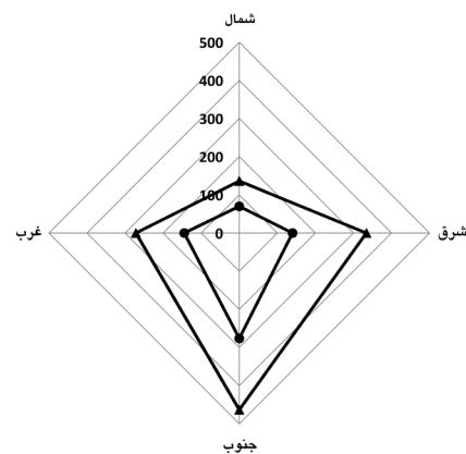
سهم تابش در شیشه دوجداره ساده (اردبیل) - سهم تابش در شیشه دوجداره ساده (استکهلم)
