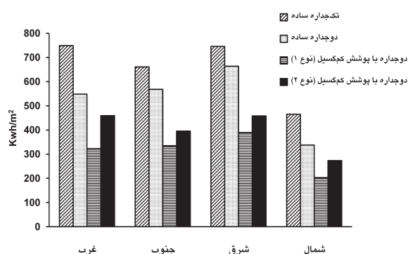
تصویر ۱۱ - بار سرمایی شیشه‌های مورد مطالعه در اوقات گرم سال در چهار جهت اصلی ساختمان.
