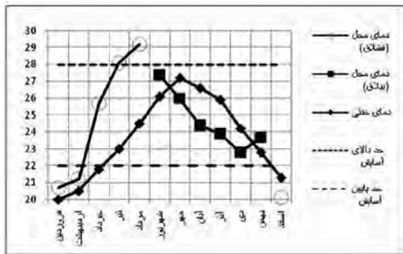
نمودار ۵- دمای حداکثر، حداقل و دمای خنثی بر اساس تئوری همیفریز و مقایسه با محدوده آسایش ایزو-۰/۷۷۳۰.
