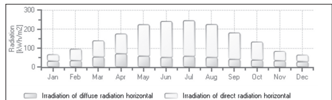
تصویر ۲- نمودار تابش خورشیدی.
