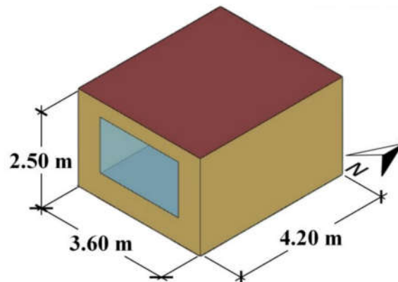
تصویر ۶. مدل شبیه‌سازی استاندارد Annex 20 برای ارزیابی عملکرد انرژی (یافت‌های پژوهش)
