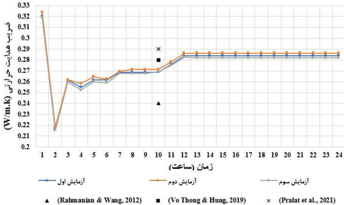
تصویر ۵. ضریب هدایت حرارتی ساعتی بلوک گچی (یافته‌های پژوهش)
