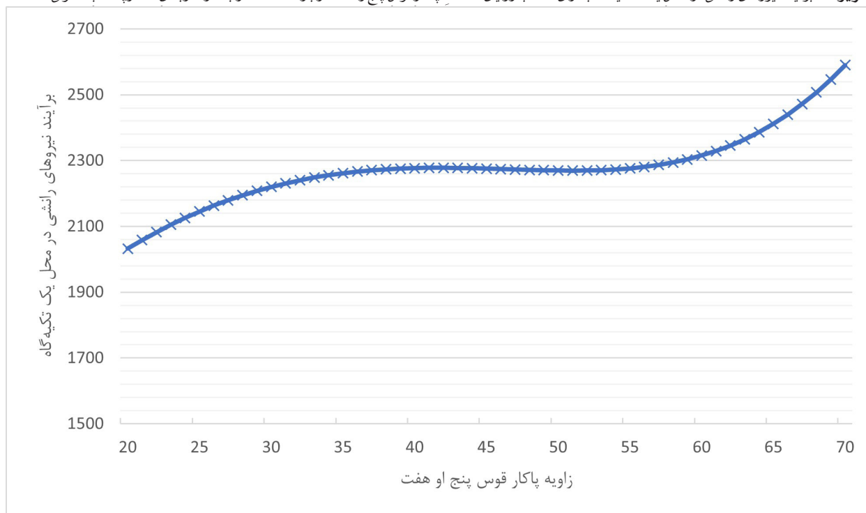
تصویر ۱۳. برآیند نیروهای رانشی در محل یک تکیه‌گاه به ازای انتخاب زوایای مختلف پاکار قوس پنج‌اوهفت در بازه ۲۰ تا ۷۰ درجه در کاربندی ۱۶ دویا، قالب شاقولی
