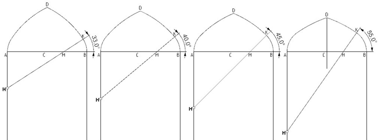
تصویر ۴. کاربردی ۱۶ دویا، قالب شاقولی در پلان (شعرباف، ۱۱۳ و ۱۶۰)
