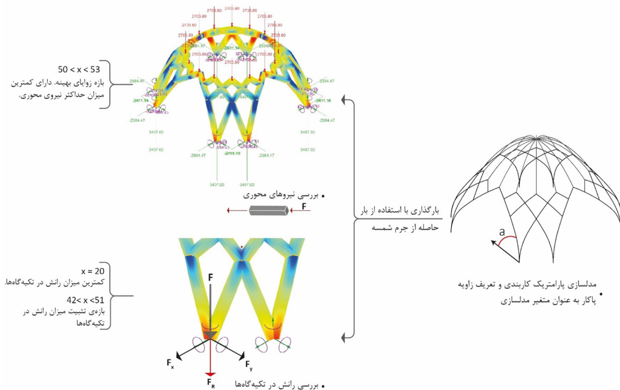
تصویر ۱۲. تصویر دو وجه اصلی بررسی شده پس از بارگذاری کاربندی‌ها با زوایای مختلف و خلاصه‌ی نتایج حاصل از آن
